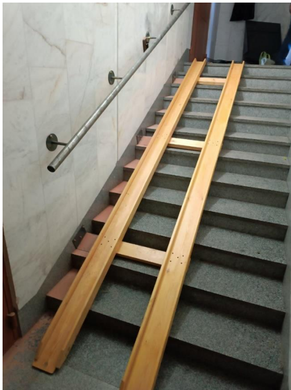
Рис. 6. Відкідний дерев'яний пандус входу до укриття.
