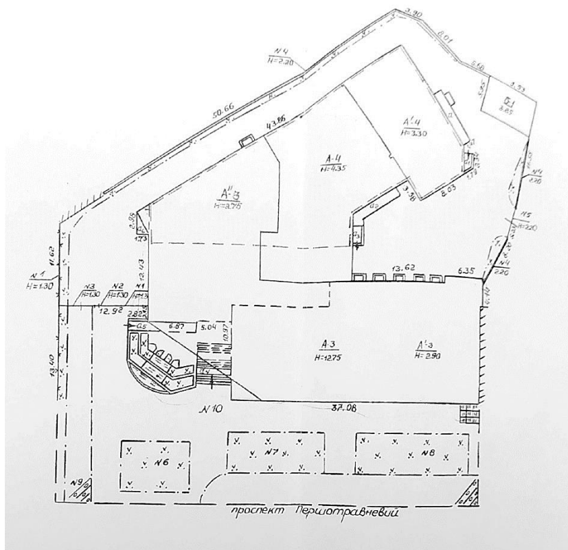
Рис. 1. Схема розташування будівлі.
